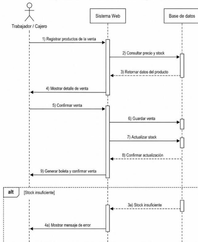
Diagrama de Secuencia – CU05: Registrar venta
