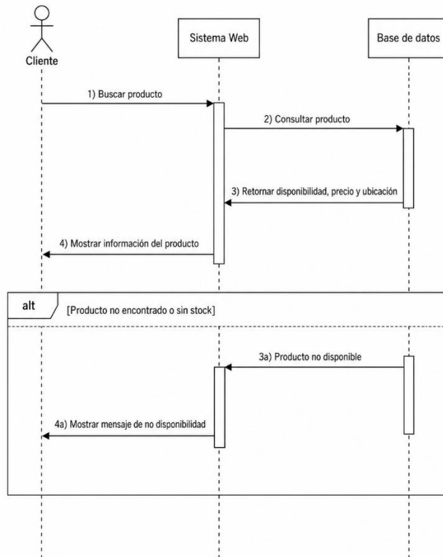
Diagrama de Secuencia – CU02: Consultar disponibilidad
